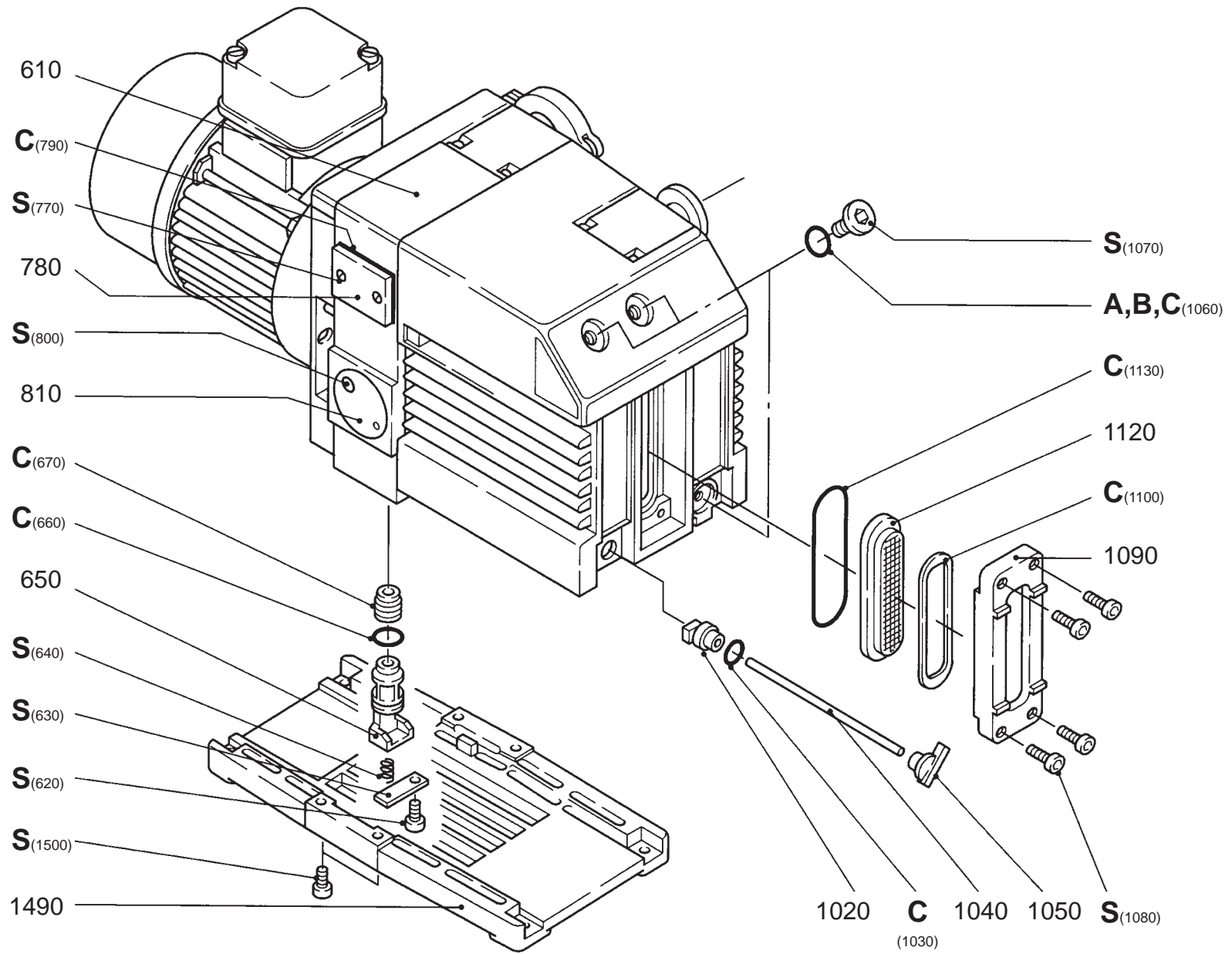
Abb./Fig. 1 TRIVAC D 16-25 B mit Gasballasteinrichtung / with gasballastvalve / avec robinet de lest d'air
