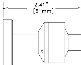
Mini Conflat™ (HPM-2002-03)
