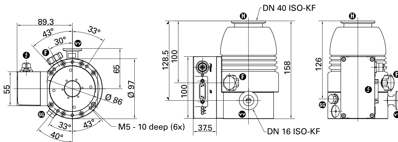
Fig. 19: HiPace 80, DN 40 ISO-KF
