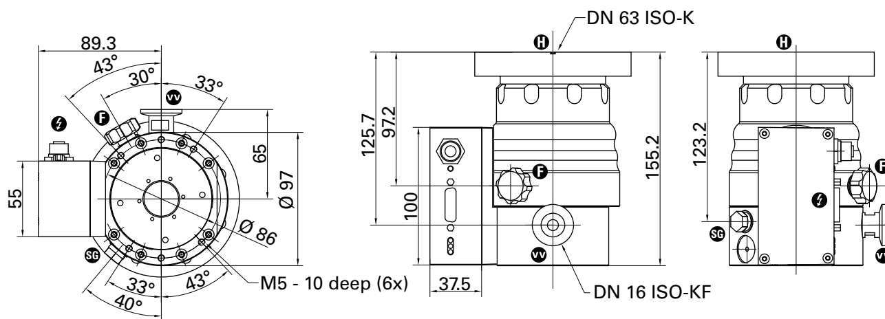
Fig. 18: HiPace 80, DN 63 CF-F
