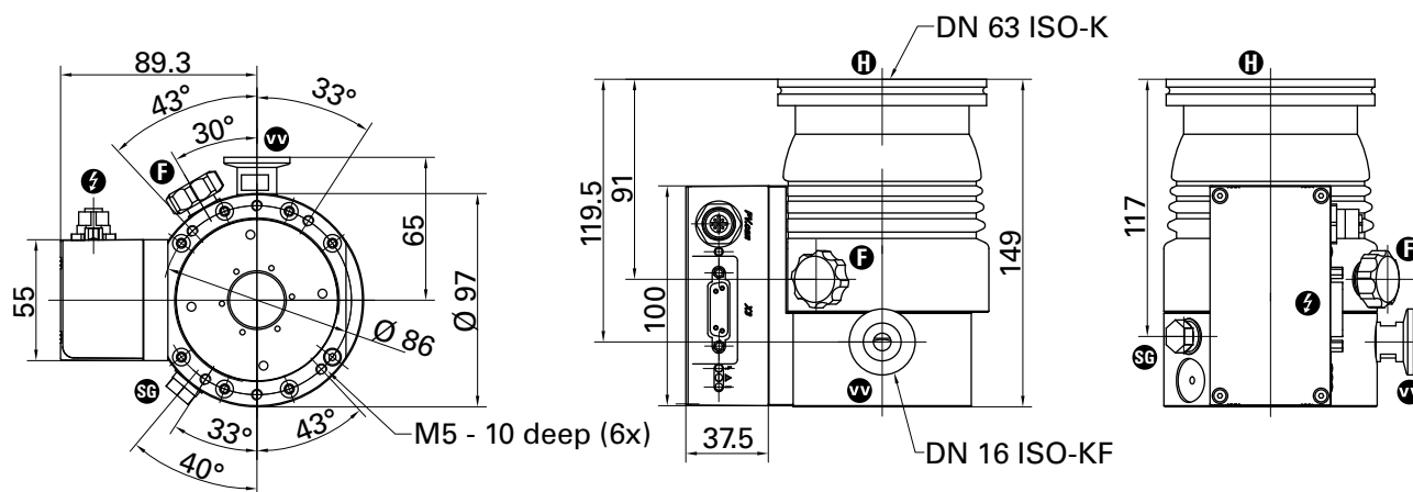
Fig. 17: HiPace 80, DN 63 ISO-K
