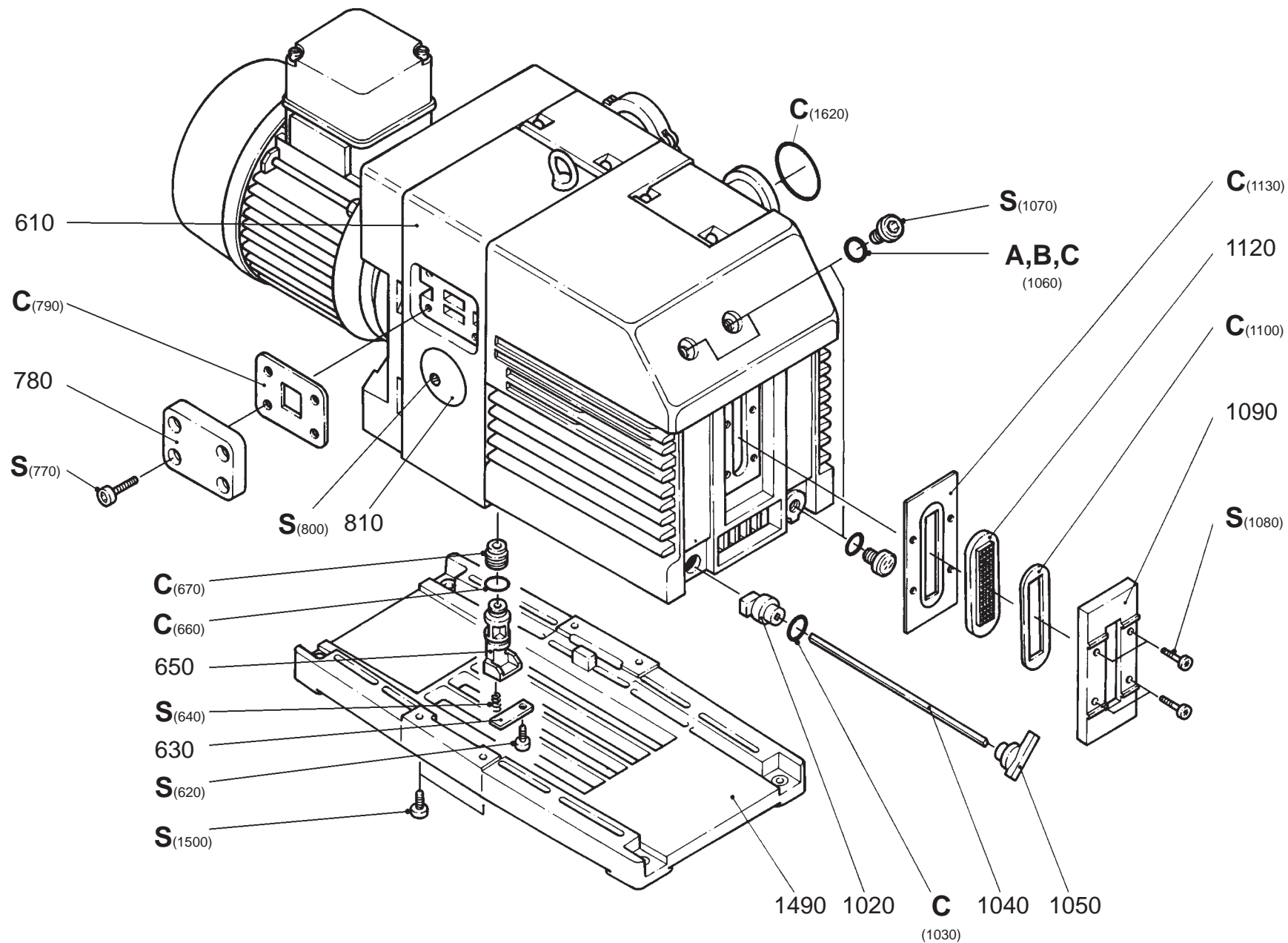
Abb./Fig. 1 TRIVAC D 40/65 B mit Gasballasteinrichtung / with gasballastvalve / avec robinet de lest d'air
