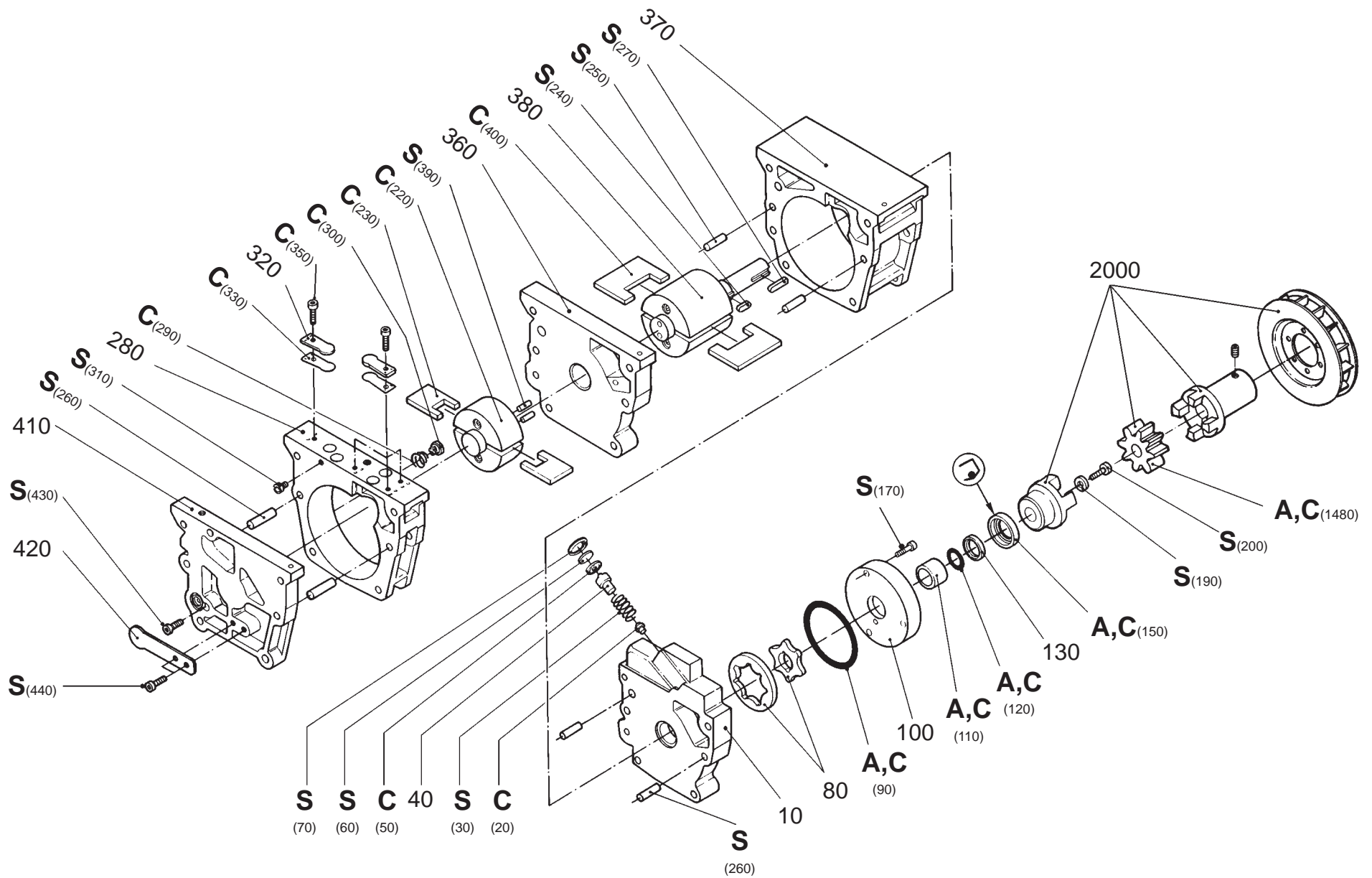
Abb./Fig. 3 Ersatzpumpmodul D 40/65 B Replacement pump module D 40/65 B Corps de pompe D 40/65 B
