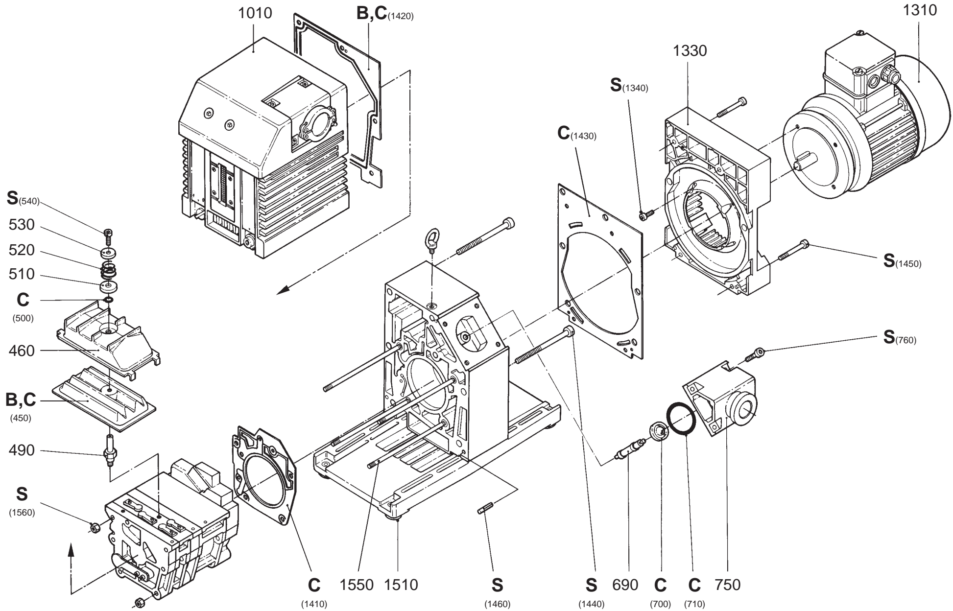
Abb./Fig. 2 TRIVAC D 40/65 B
