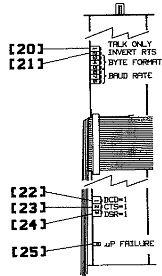
Fig. 4.1 RS-232 Module Top View
